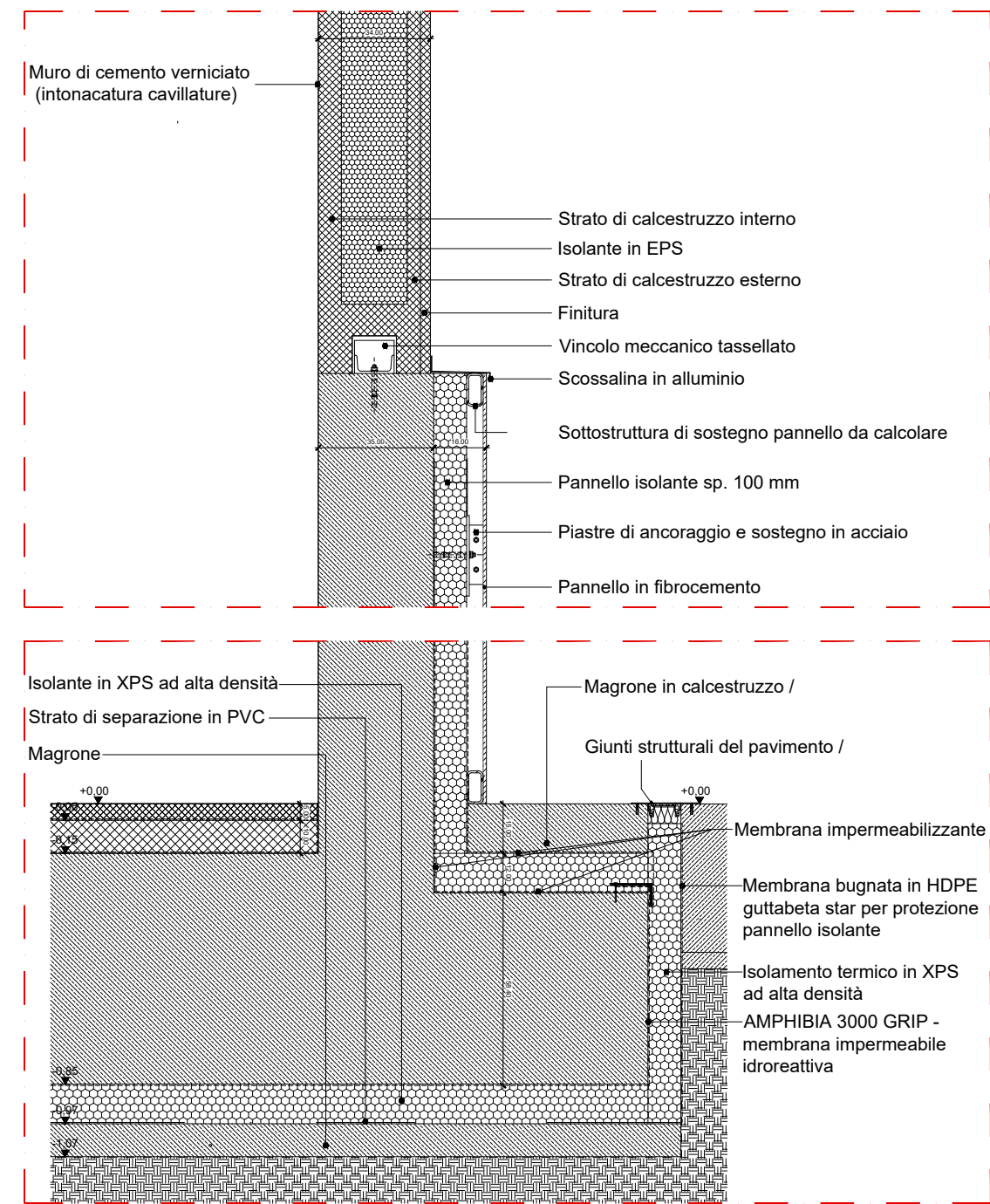
Dettaglio attacco a terra Scala 1:20
