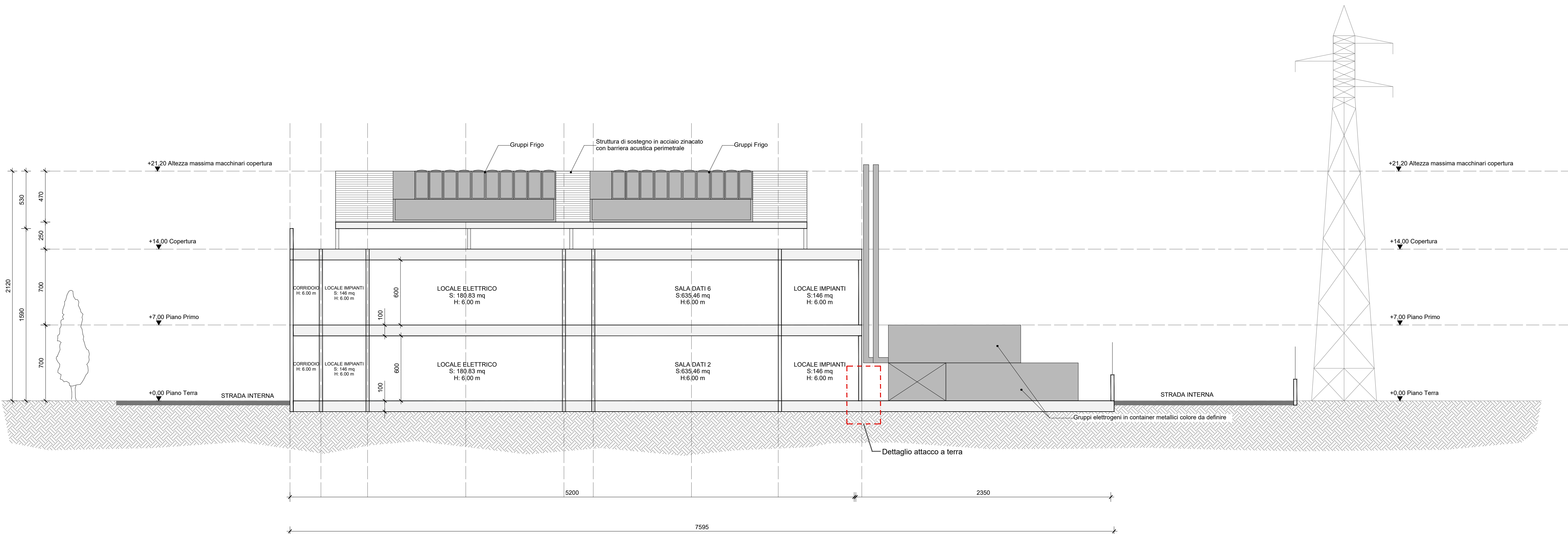
Sezione A-A
